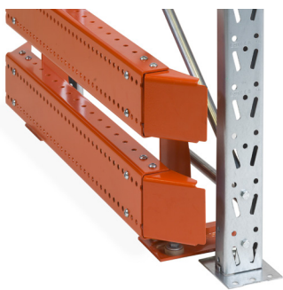
Päädyn törmäyssuoja - päädyn suojaukseen. Korkeus 400 mm.
