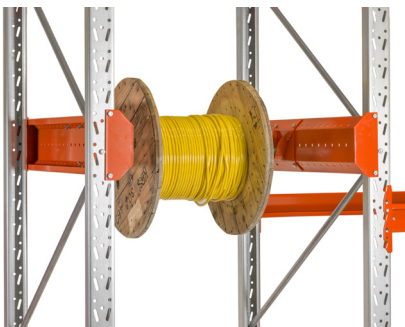
Kelan ripustus - itselukittuvalla akselilla. Kela säädettävissä sekä sivusuunnassa akselilla että syvyysuunnassa. Välikköpituus 950 ja 1350 mm.
