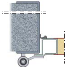
U - 60 x seinäpaksuus x 5 mm
