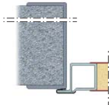
U - 60 x seinäpaksuus x 5 mm
