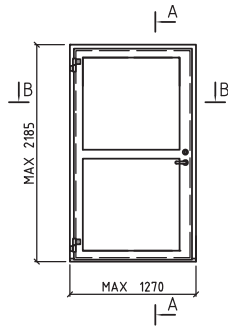
ENKELFLYGLIG SÄKERHETSDÖRR SS-EN 1627:2011 RC 3
