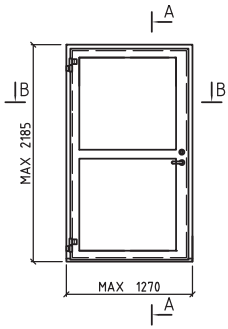
ENKELFLYGLIG SÄKERHETSDÖRR SS-EN 1627:2011 RC 2
