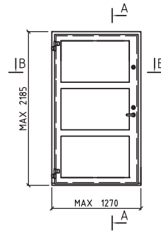
ENKELFLYGLIG SÄKERHETSDÖRR SS-EN 1627:2011 RC 4
