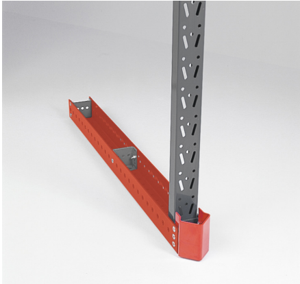
Vahvistettu alaohjausprofiili haarukatrukkiohjaimella.
