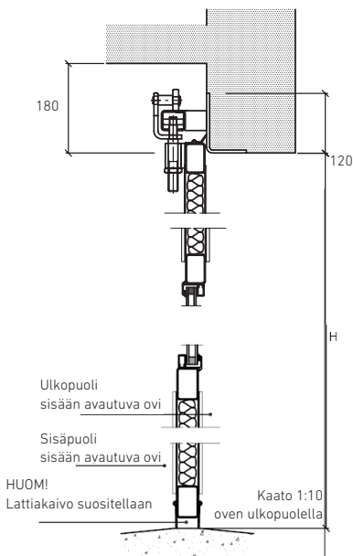
Kantava ohjaushela Yli 4,5 m leveä ovi
