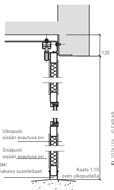
Ohjainhela Enintään 4,5 m leveät ovet
